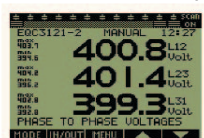
Digits Display
